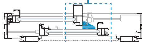
Bottom stopper
